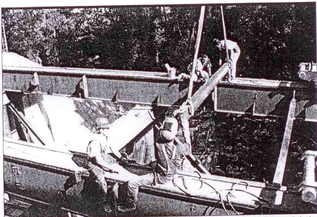
ÚTZÁR A 44-ES FŐÚTON. A szolnoki oldalon szerdára, illetve mára virradó hajnalban a helyükre emelték az épülő tiszaugi új közúti híd beton tartógerendáit. A munkálatok idejére mindkét nap átmenetileg teljesen lezárták a 44-es főút forgalmát. Felvételünkön az összeszerelt hídelemek átcsúsztatására szolgáló sínpályát készítik.
