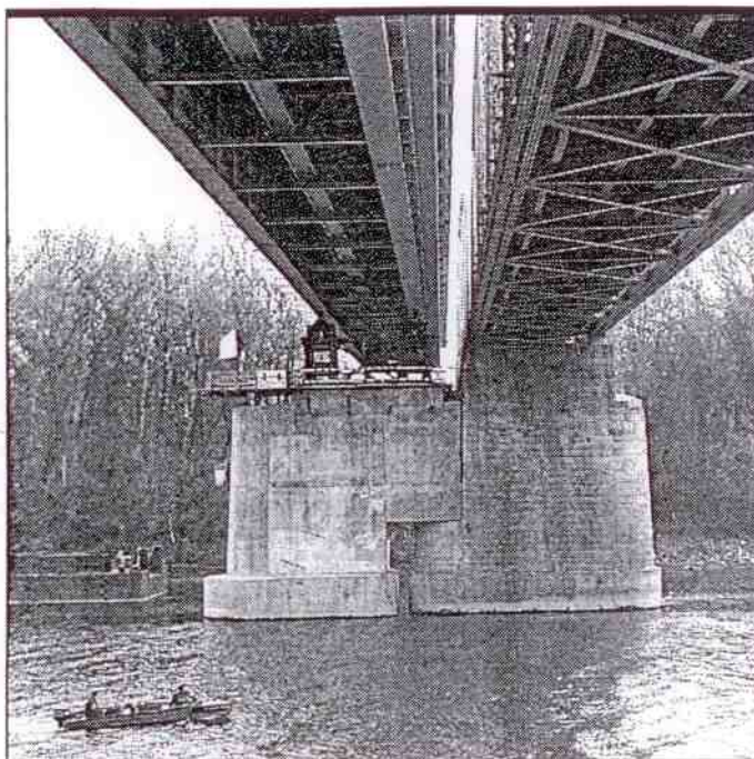
LEÁLLT A HÍDÉPÍTÉS. Az év végi ünnepek idejére leállt a tiszaugi közúti híd építése. A földmunkák többsége elkészült. A két részből álló híd szerkezet hosszabbik fele is elérte már a Tisza bal oldali partját.
