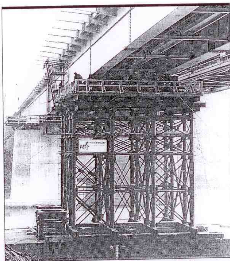
EGY DARABBAN A HÍDTEST. Péntek óta egy darabban van az épülő tiszai közúti híd úgynevezett felszerkezeti része. A több mint 300 méter hosszú hidat október 23-án tervezik átadni. FOTÓ: SZ. A.
